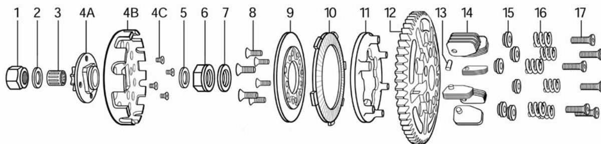
HORSTMAN CLUTCH
